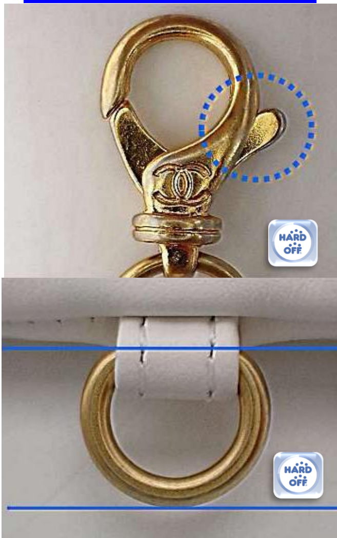
基準内のフックとポーチD管
